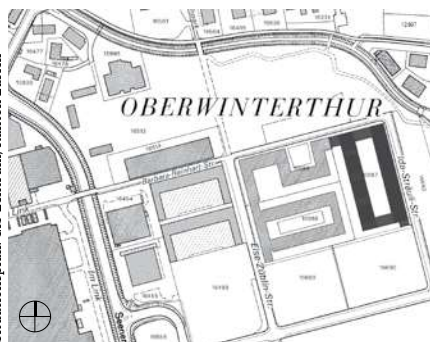
Situationsplan: GIS-Zentrum, Kanton Zürich
